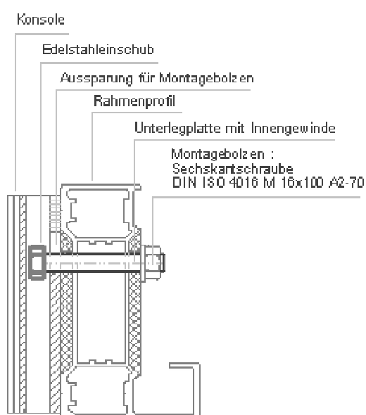
MONTAGE KONSOLE-RAHMENMONTAGEBOLZEN
