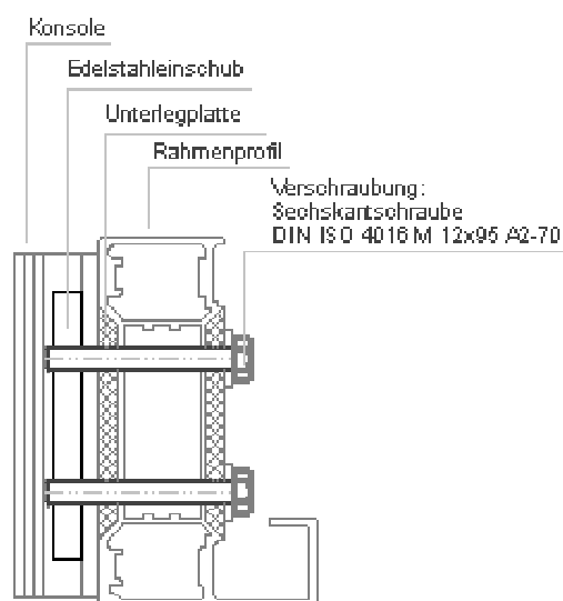
VERSCHRAUBUNG KONSOLE-RAHMEN
